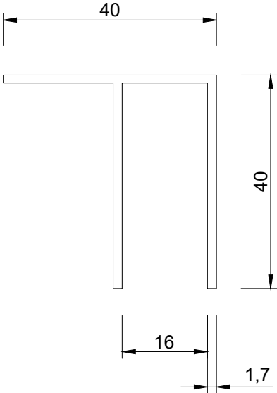
Doorsnede
