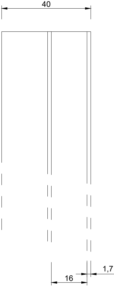
Zijkant
